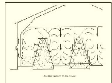
鶏舎内の空気の動き
