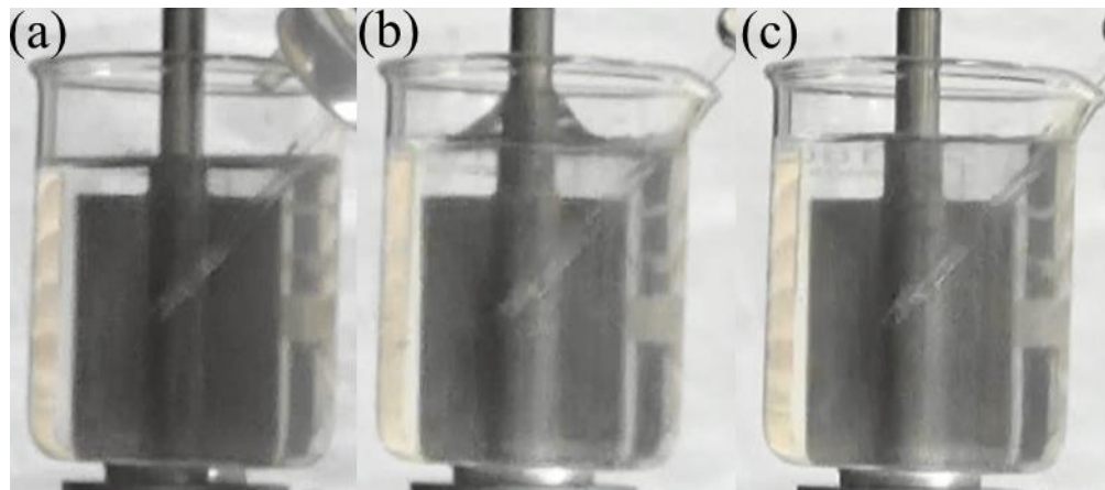
図 1 本研究で観察された化学反応前後の流体物性では予測できない高分子溶液反応流 (a)ビーカー内で 150 rpm で攪拌翼により攪拌されている pH = 11 に調製された部分的に加水分解されたポリアクリルアミド水溶液 (分子量 5-6 百万、濃度 1 wt%) 90 mL に、(b)10 mL の硝酸アルミニウム水溶液 (濃度 0.01 M) を注ぐと、ワイゼンベルグ効果が生じる。(c) 一定時間が経過すると、ワイゼンベルグ効果は消失する。
