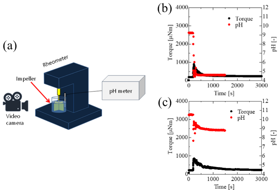
図 2 (a)攪拌トルク・pH 同時測定装置図 攪拌トルクはレオメーターにより、pH は pH メーターにより測定した。(b)(c)攪拌トルク・pH 同時測定結果 硝酸アルミニウム水溶液は t=180 s に添加した。ワイゼンベルグ効果の出現・消失に対応して攪拌トルクが一時的に増加した。ワイゼンベルグ効果の一時的な出現及び消滅が発生するのは、硝酸アルミニウム水溶液添加直後に(b)pH が大きく下がる場合と、(c)pH がほとんど変化しない場合の二通りの場合があった。
